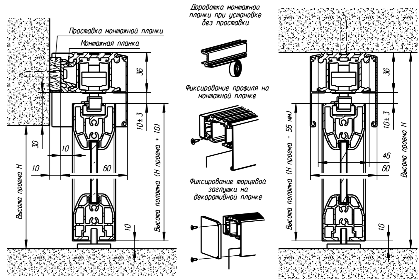
Схема крепления к стене/потолку (2-1)
