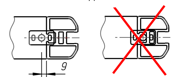
Схема крепления к потолку (2-4)
